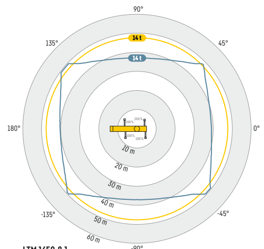
LTM 1650-8.1 54 m 100% 560° 95 t
