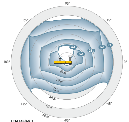
LTM 1650-8.1 54 m 100% 560° 65 t
